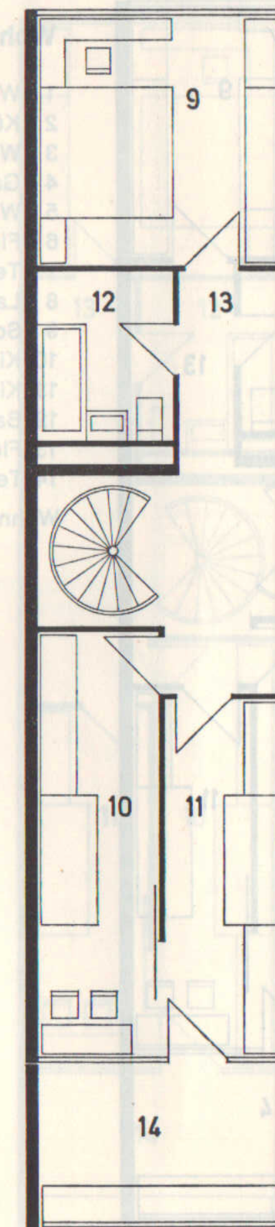
Ebene 04 (2. OG)
