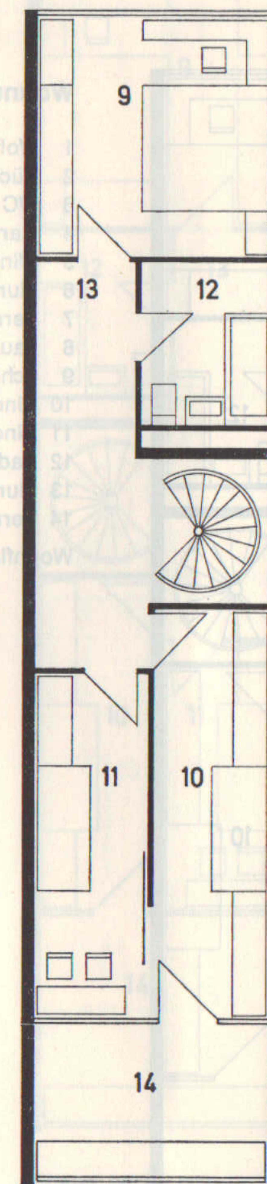
Ebene 04 (2. OG)
