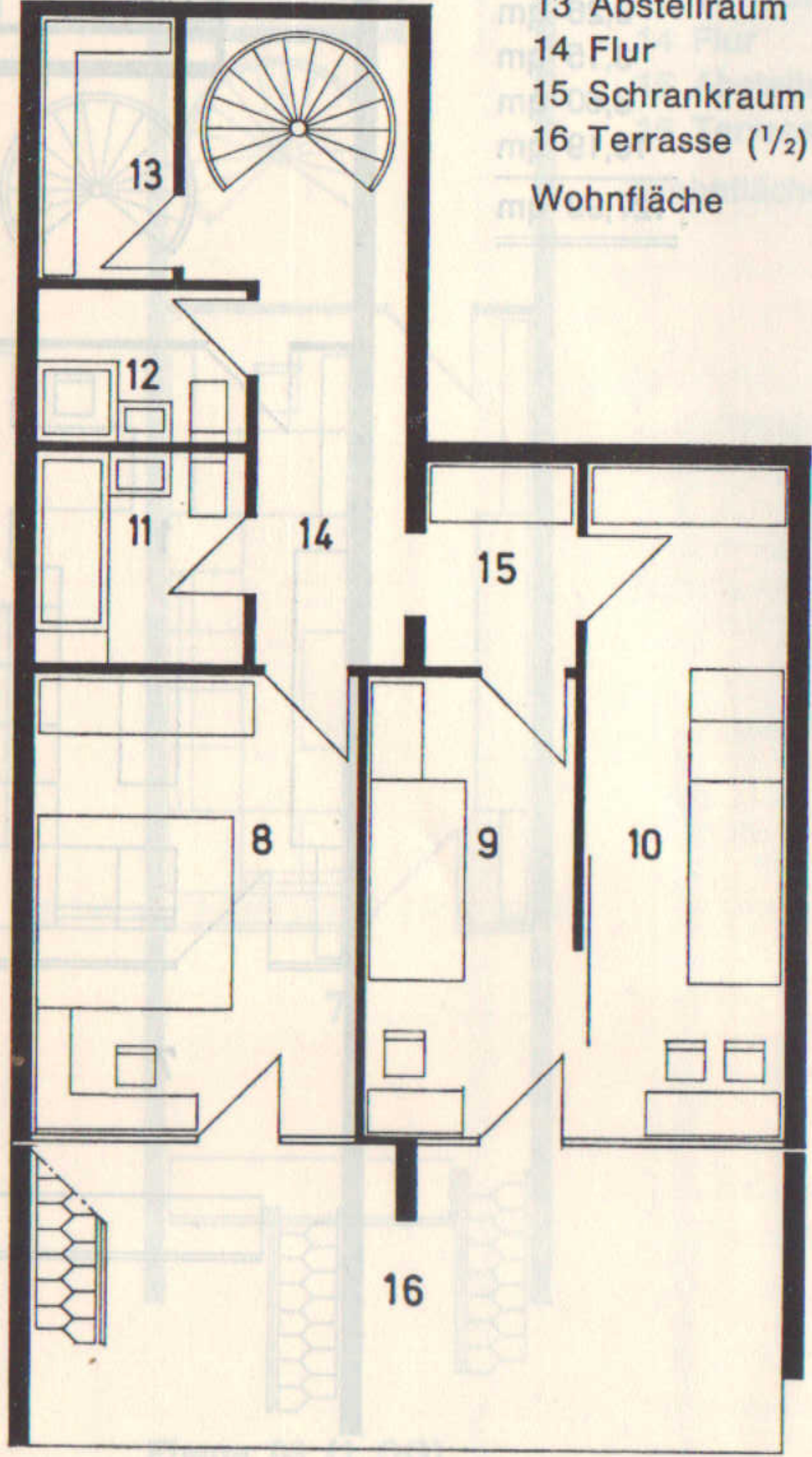
Ebene 02 (EG)
