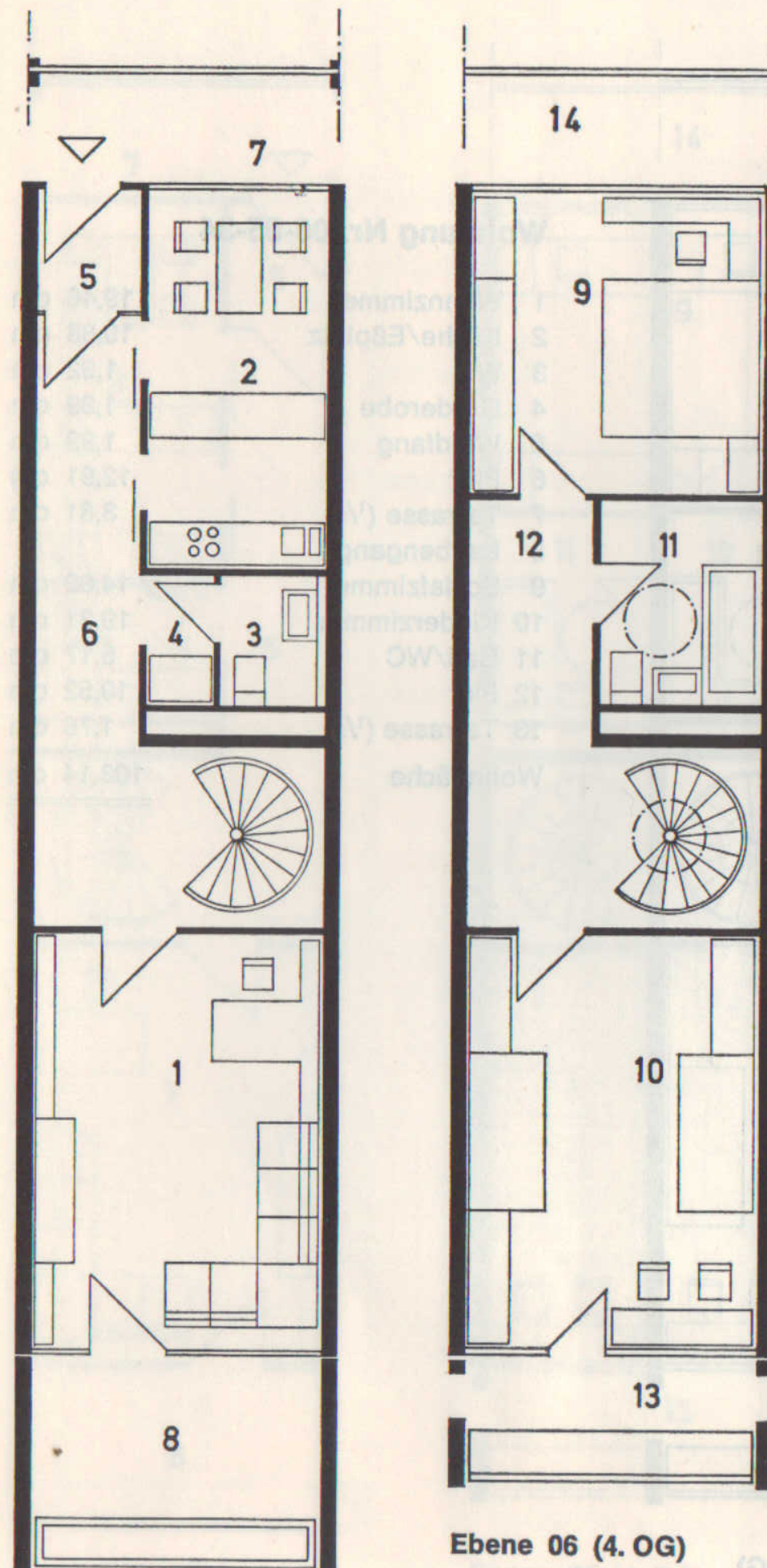
Ebene 05 (3. OG), Wohnungseingang
