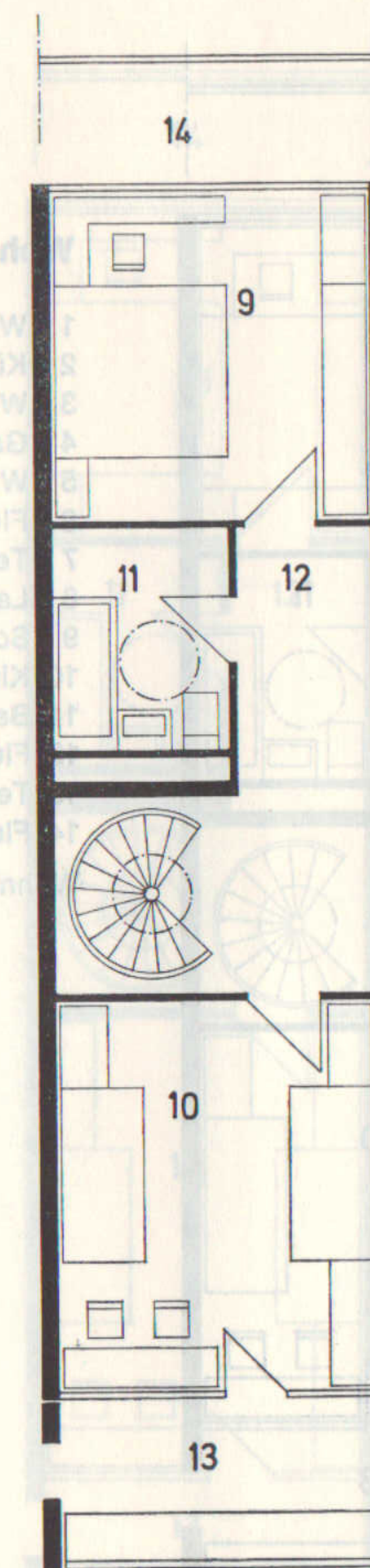
Ebene 06 (4. OG)
