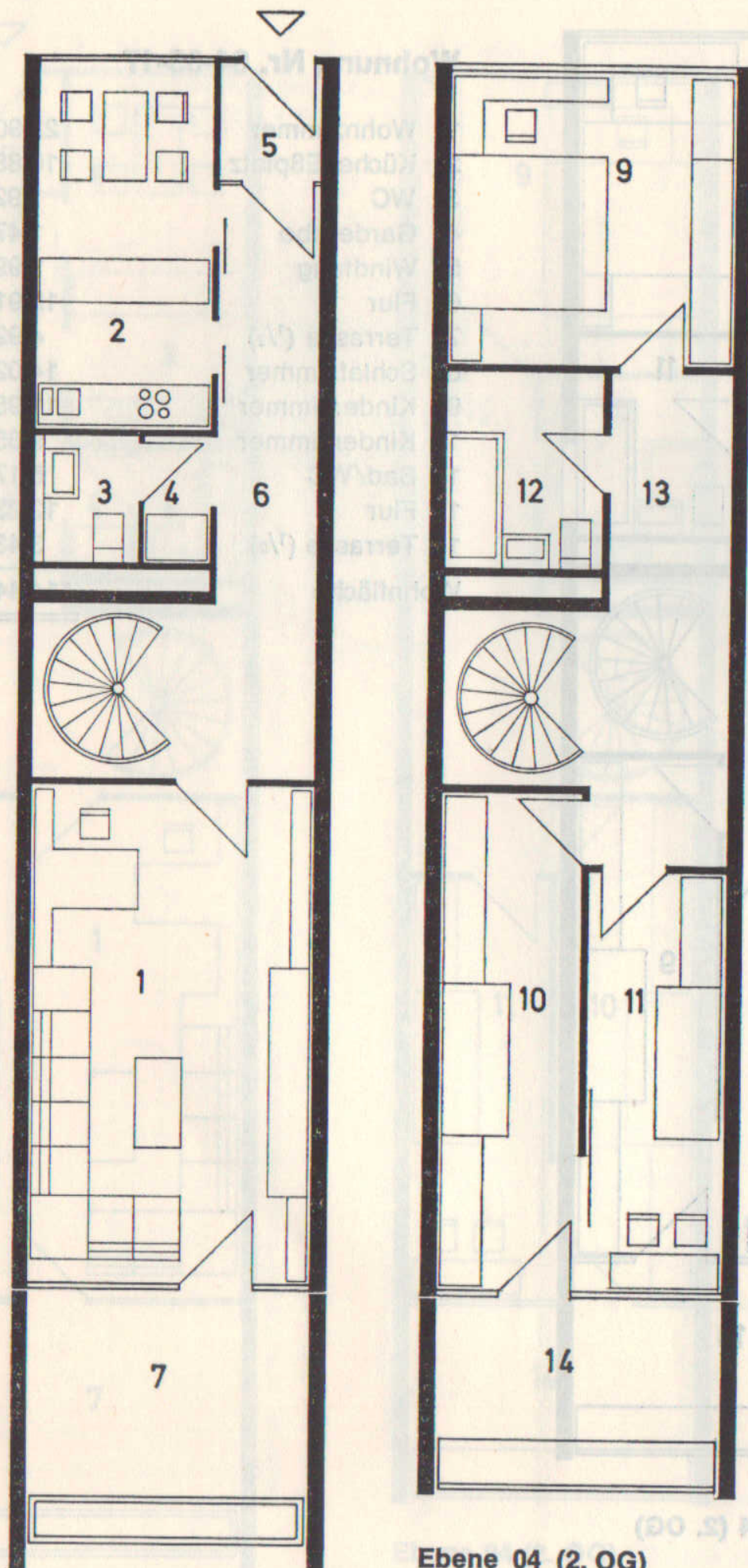
Ebene 03 (1. OG) Wohnungseingang
