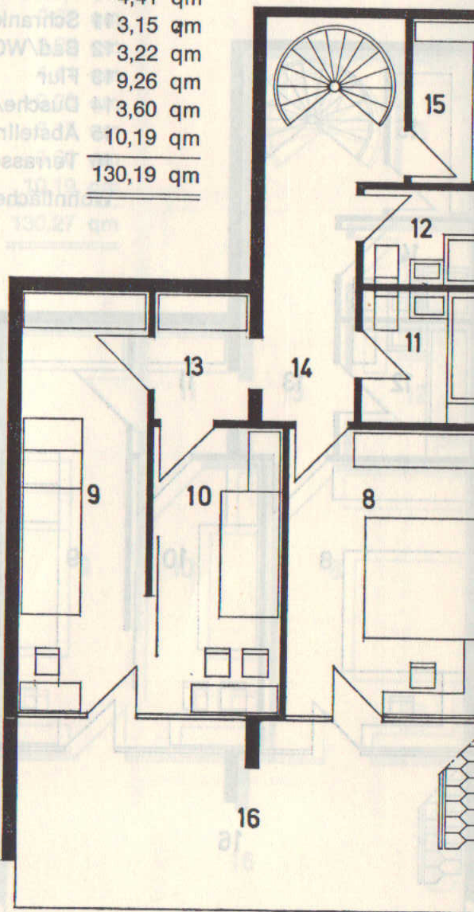
Ebene 02 (EG)
