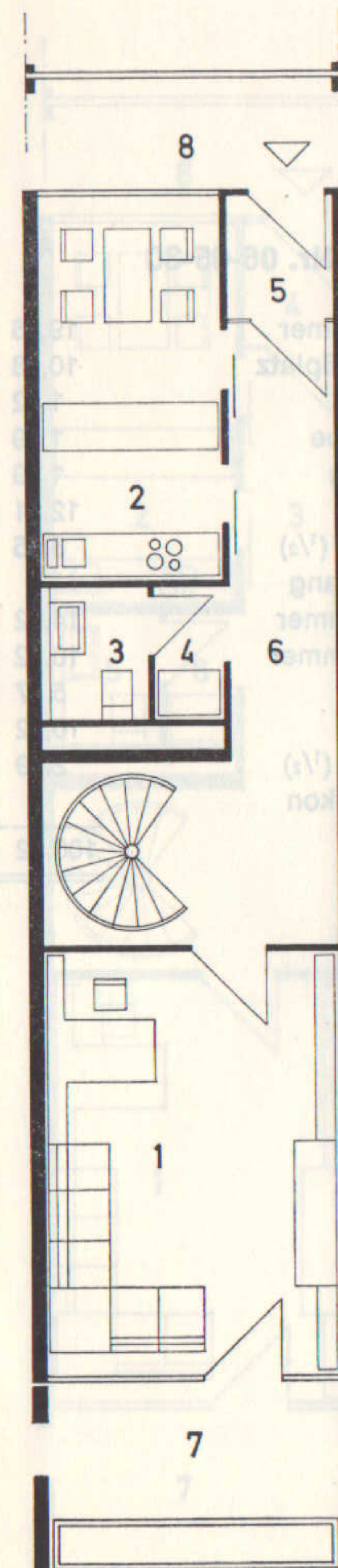
Ebene 05 (3. OG) Wohnungseingang
