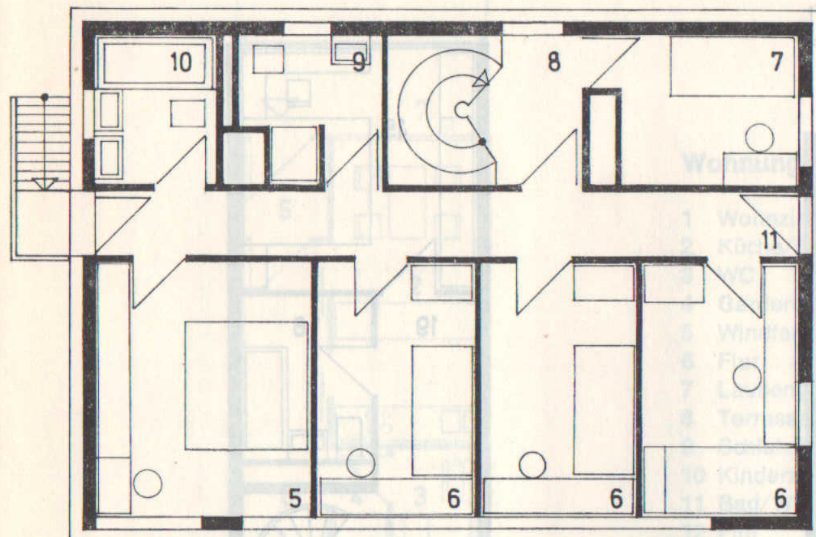
Ebene 11 (8. OG)
