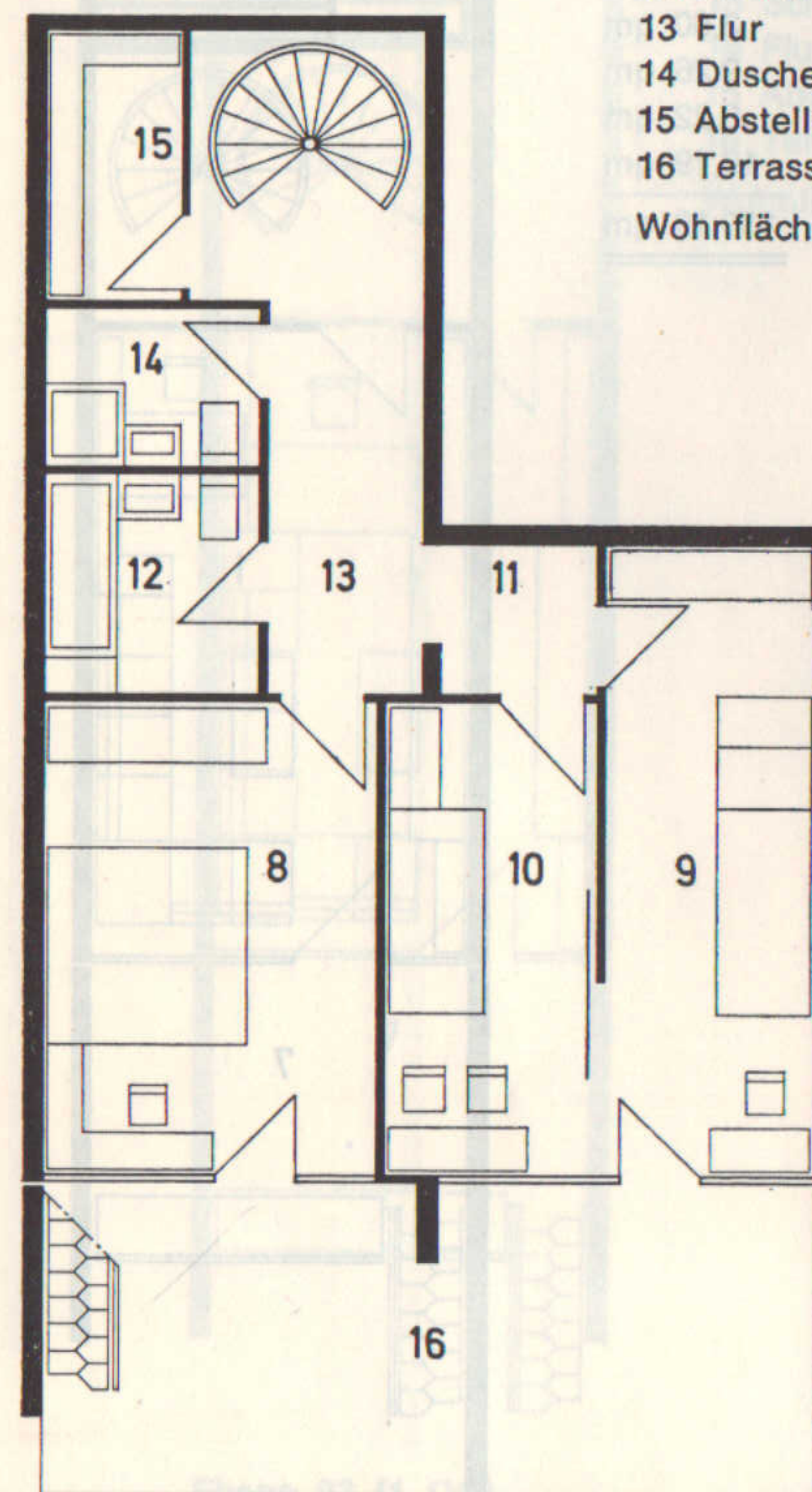
Ebene 02 (EG)
