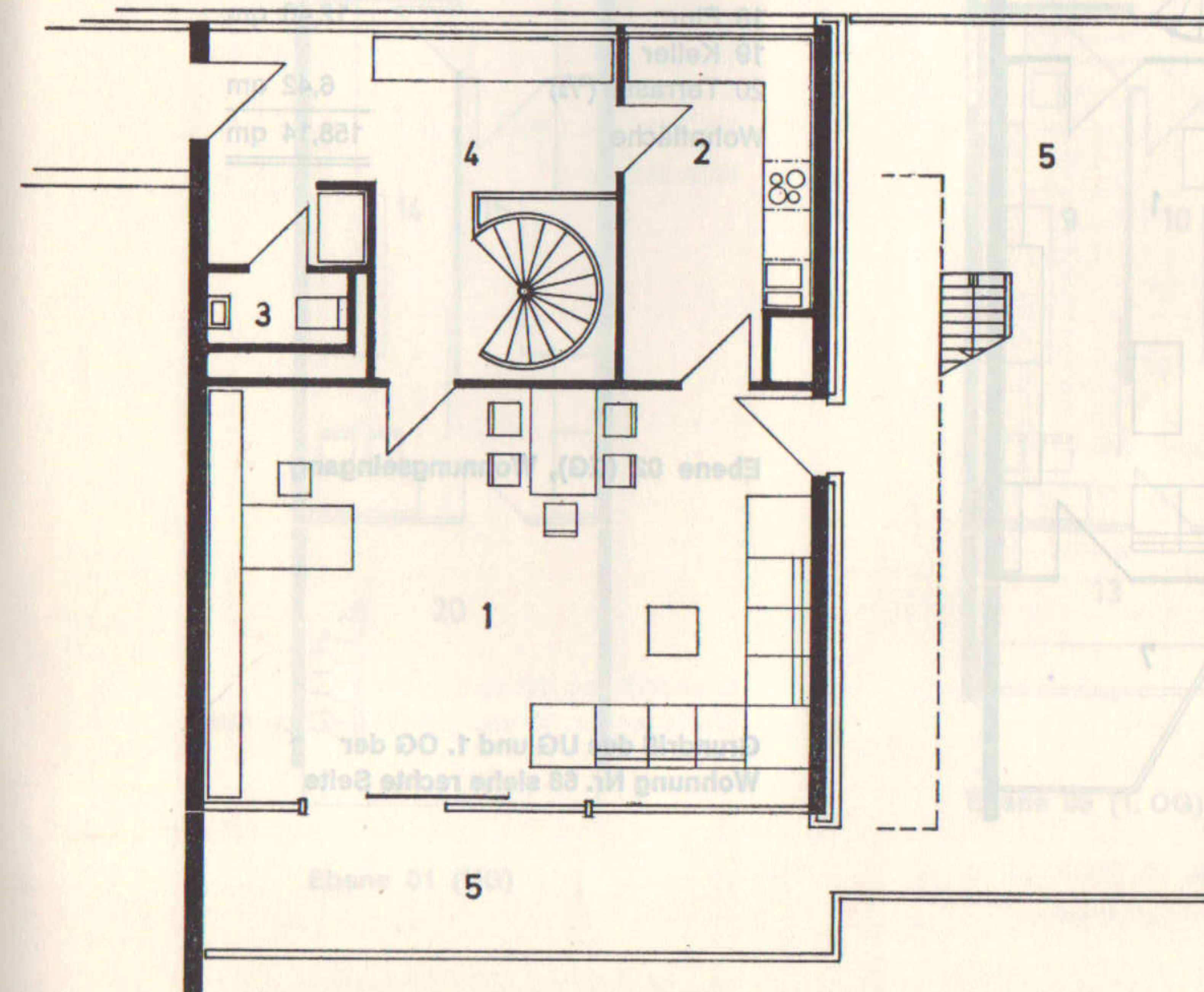
Ebene 12 (9. OG), Wohnungseingang
