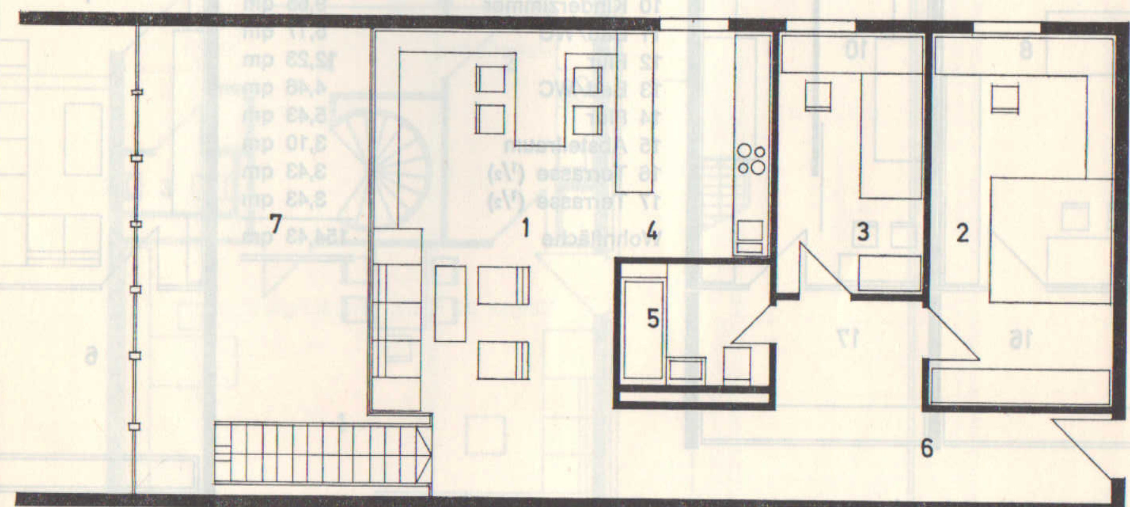
Ebene 02 A (1. UG), Wohnungseingang
