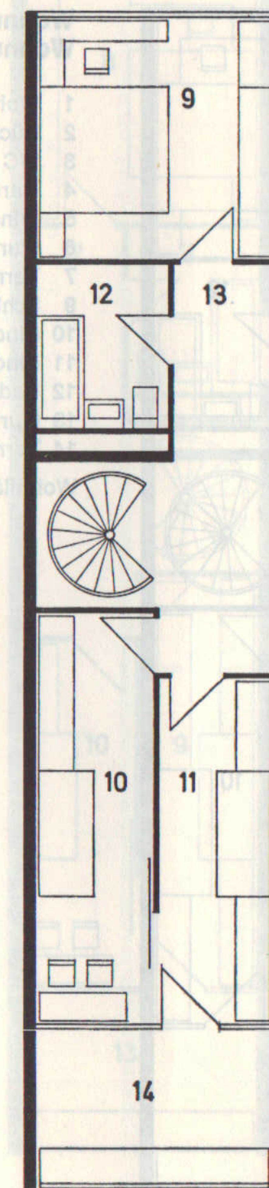
Ebene 04 (2. OG)
