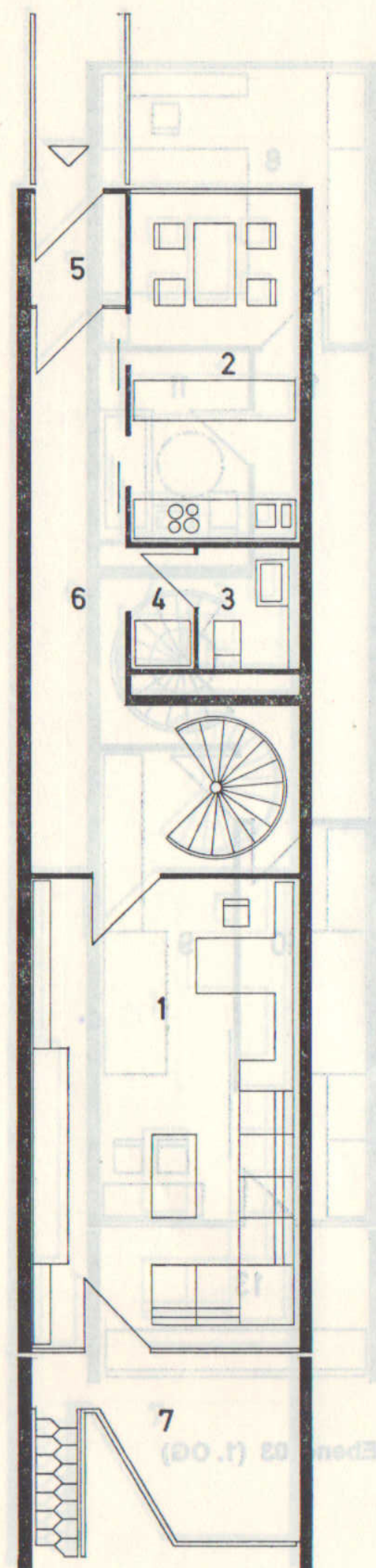
Ebene 02 (EG) Wohnungseingang
