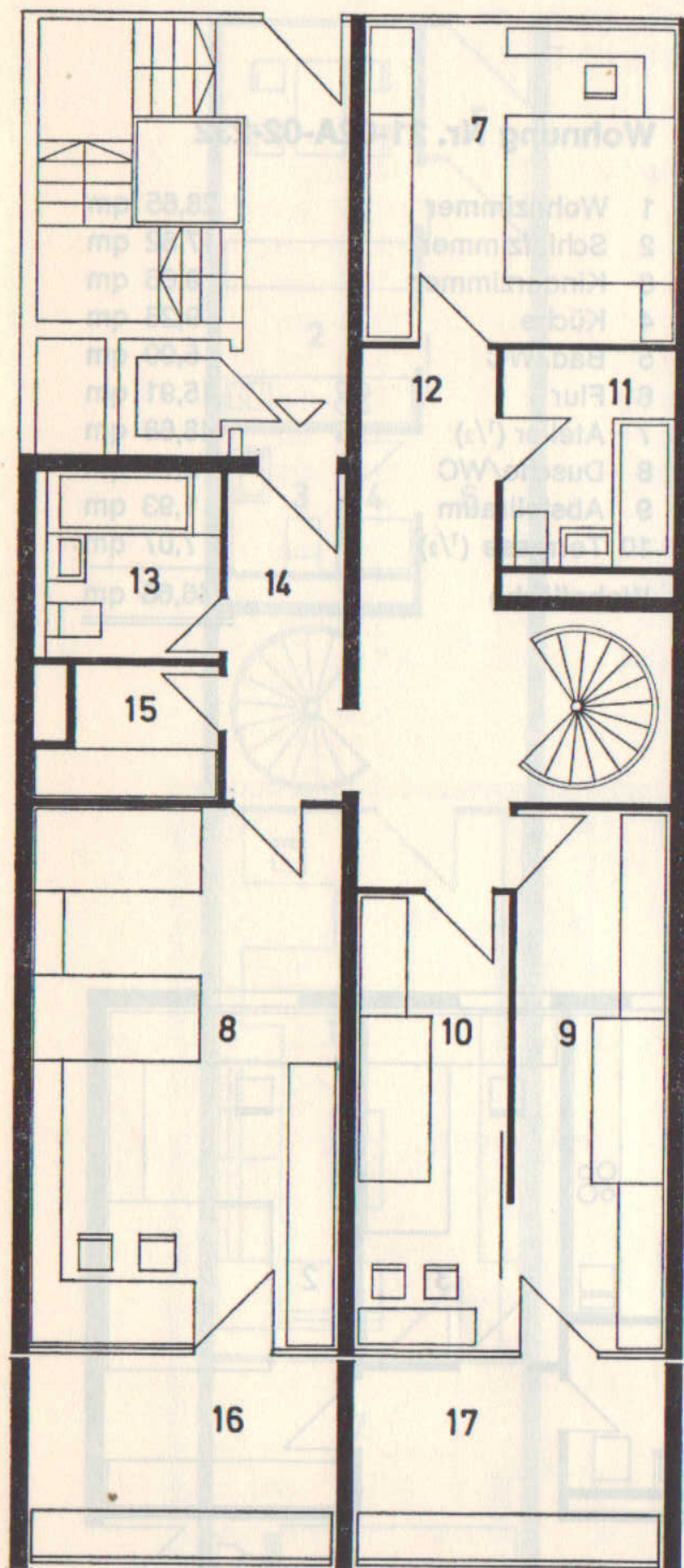
Ebene 04 (2. OG), Nebeneingang
