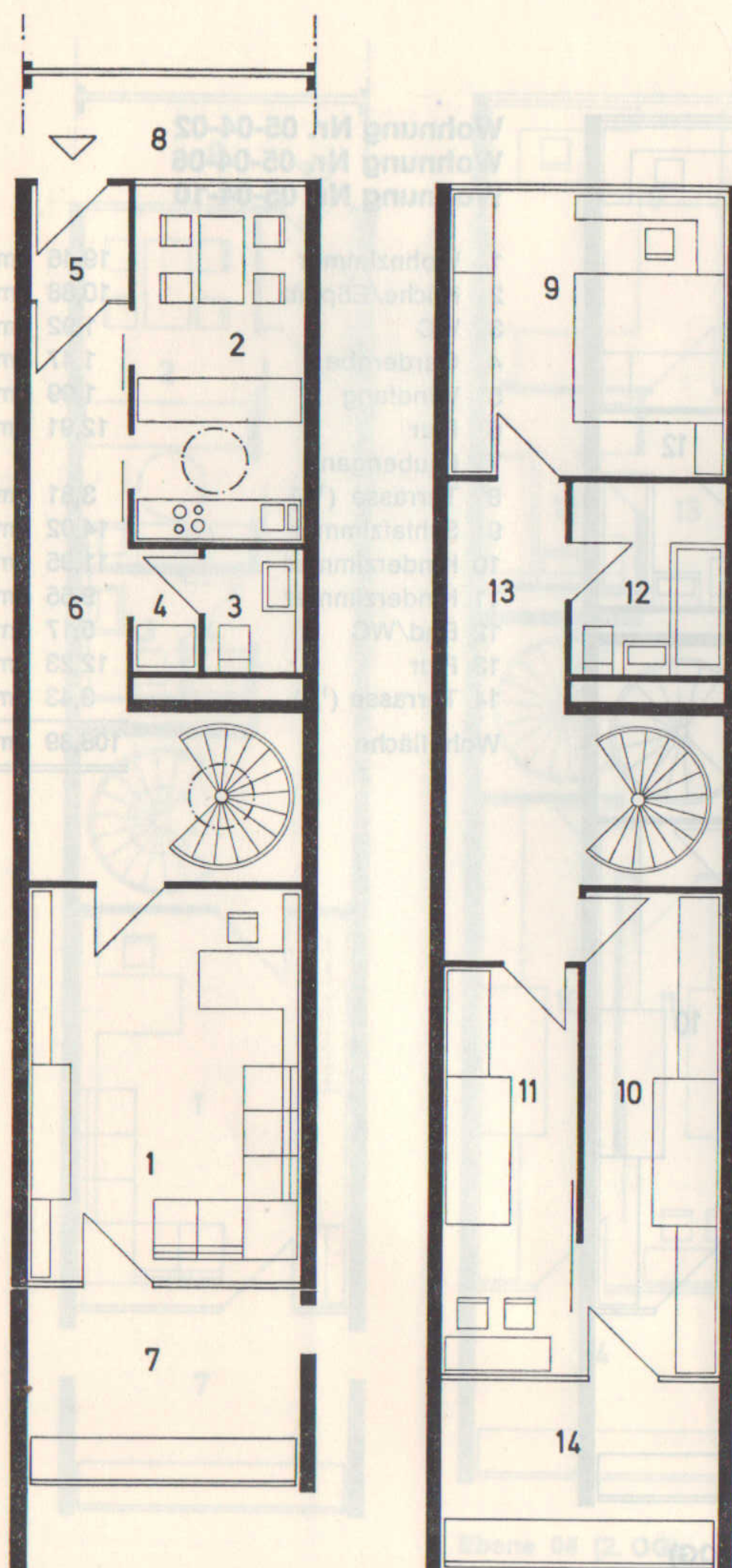
Ebene 05 (3. OG) Wohnungseingang
