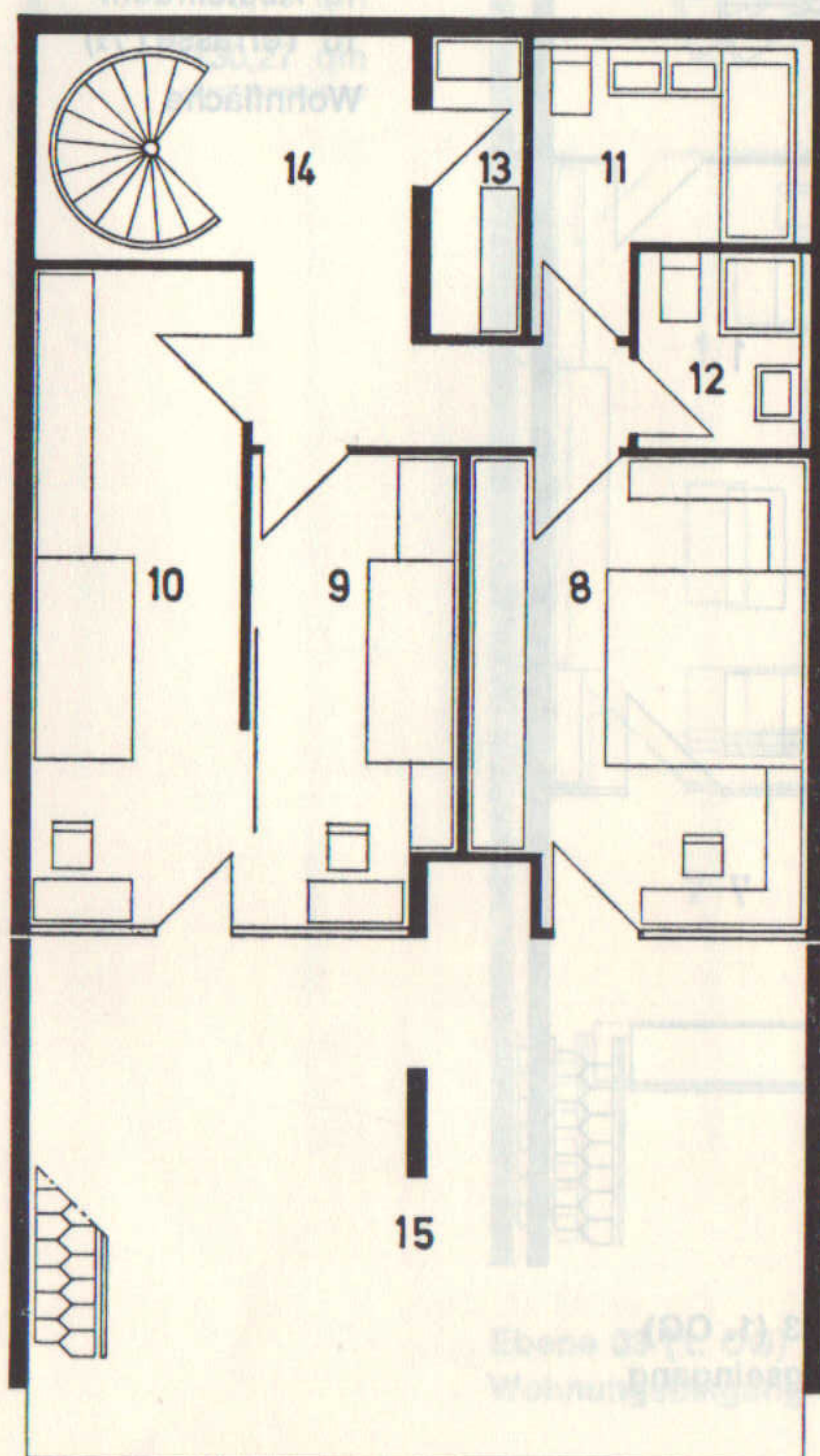
Ebene 02 (EG)
