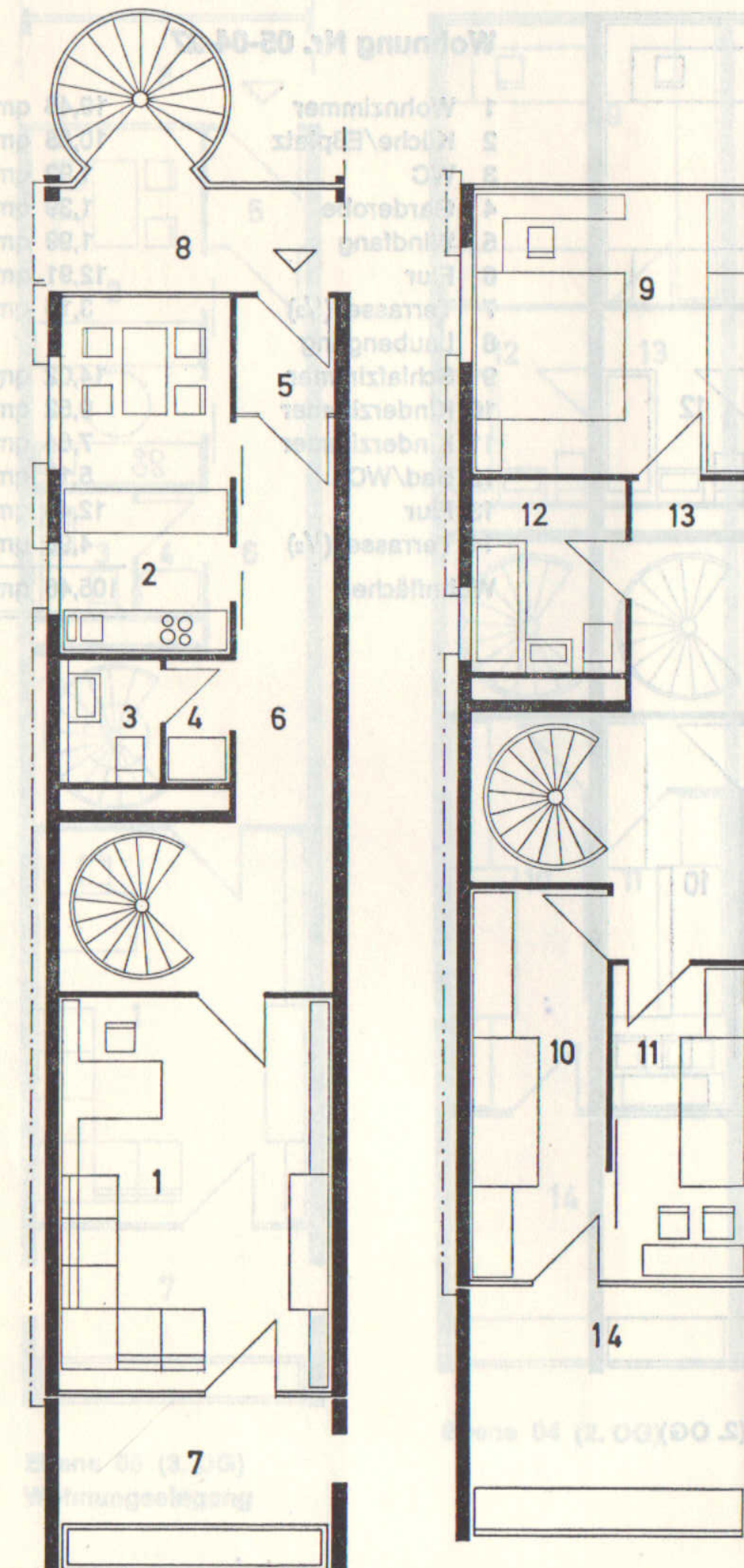
Ebene 04 (2. OG)
