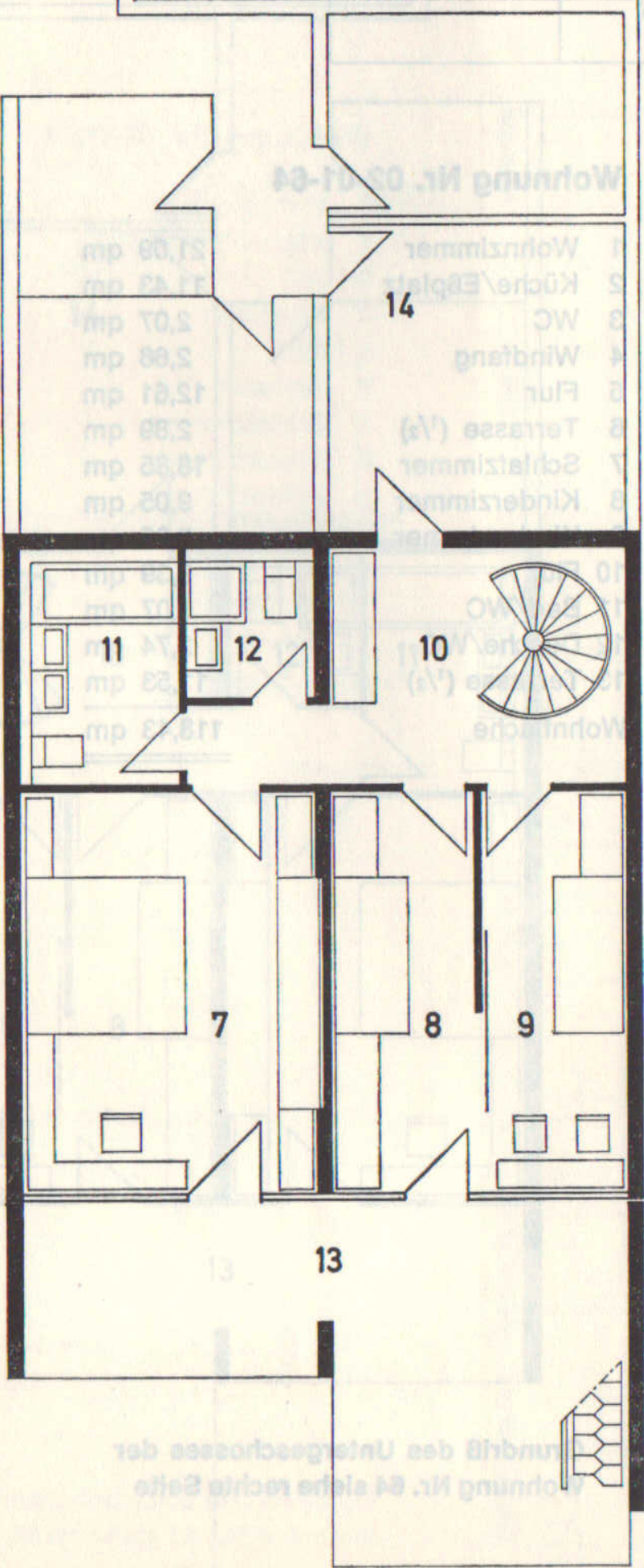
Ebene 01 (UG), Nebeneingang
