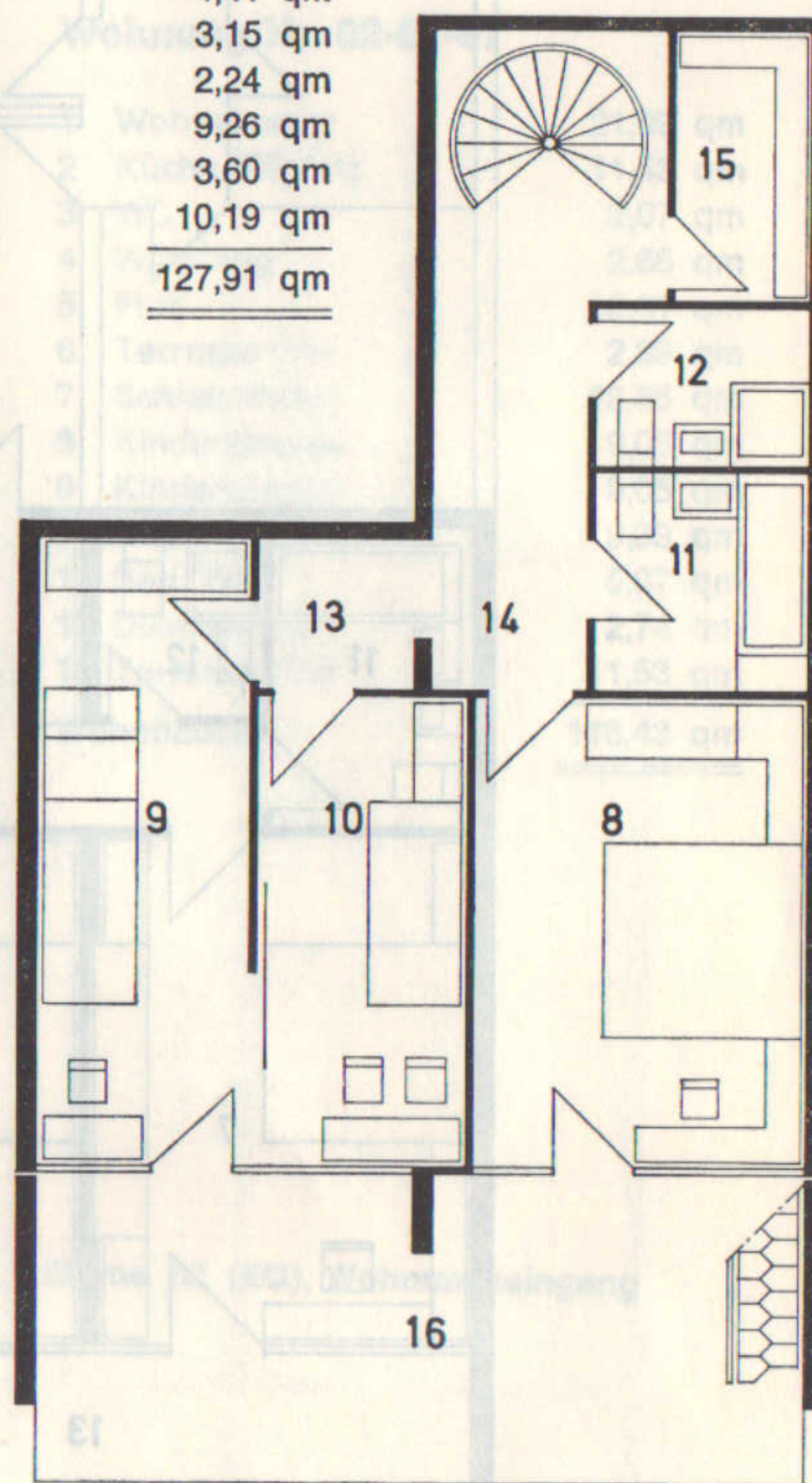
Ebene 02 (EG)
