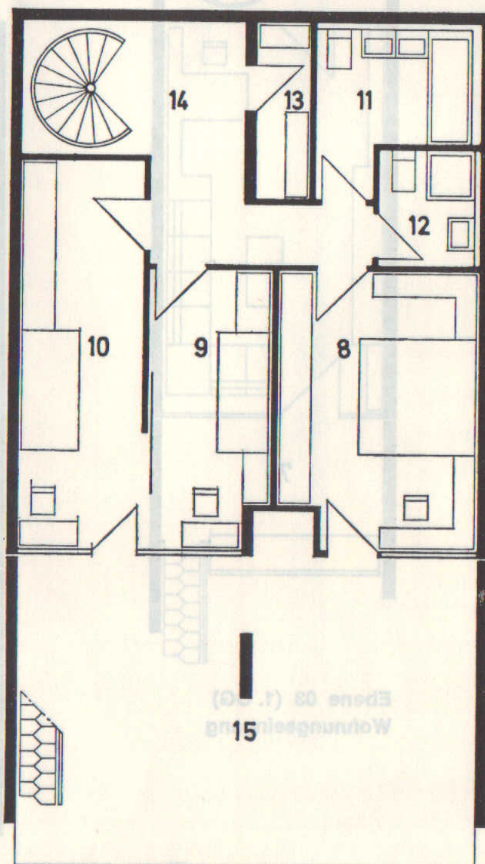
Ebene 02 (EG)
